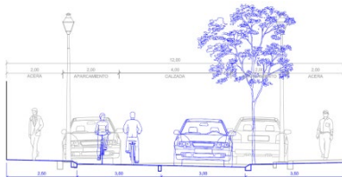
Sección propuesta / Itinerarios principales vehículos / Señalización escolar
